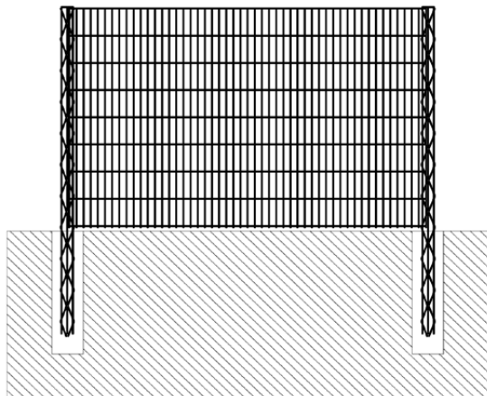
Рис. 2 Установка на грунт
