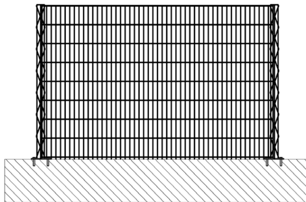
Рис. 3 Установка на твердое основание
