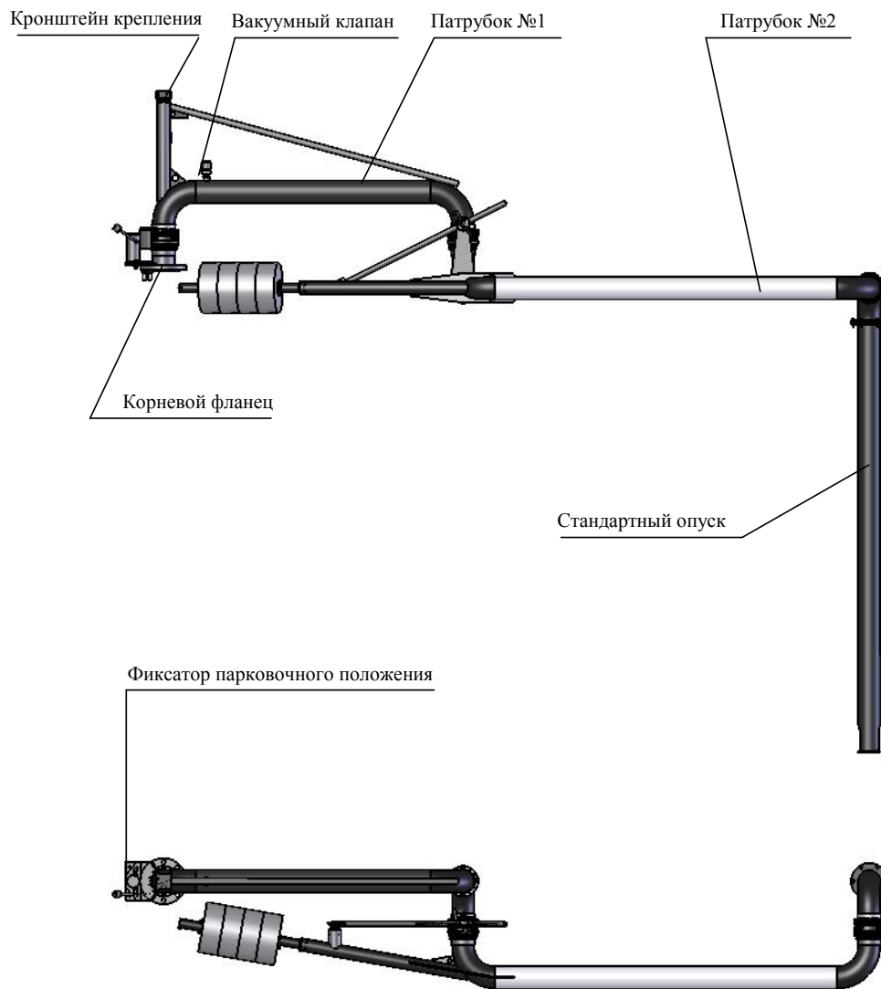
Рис. 1. Конструкция стойки верхнего налива ОСН-СВН-100-Н-А-4-НН.
